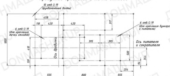
Схема расположения фундаментных болтов, места поступления продуктов дробления и точки отходов
