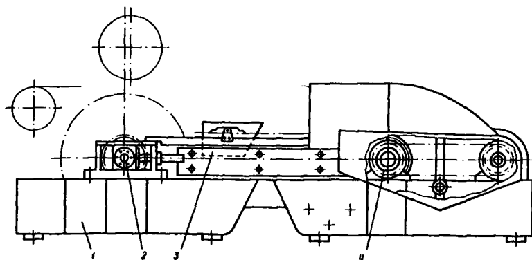
Черт.6. Пробоотборник ковшовый типа ПК;
