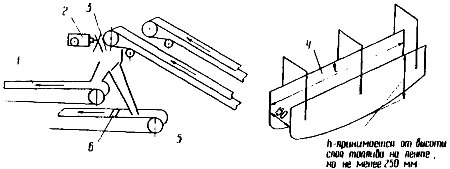
Черт.15. Схема контрольного отбора проб с остановленной ленты конвейера при приемочных испытаниях пробоотборника:
