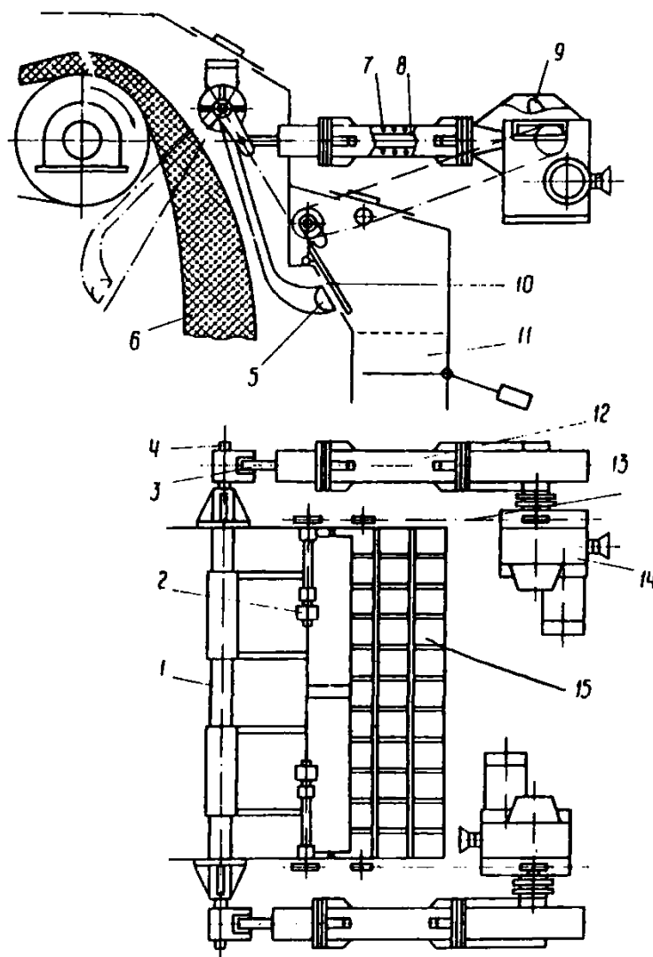
Черт.5. Автоматический отборник АО2-ВТИ:
