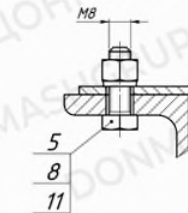
Г-Г (1 : 1)
