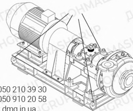
Схема строповання
