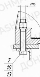
Д-Д (1 : 2)
