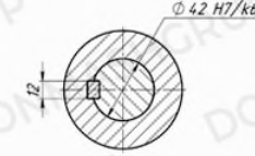
Ж-Ж (1 : 2)
