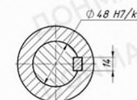
Е-Е (1 : 2)
